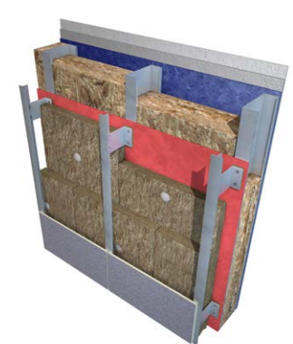
Steel frame - double layer
