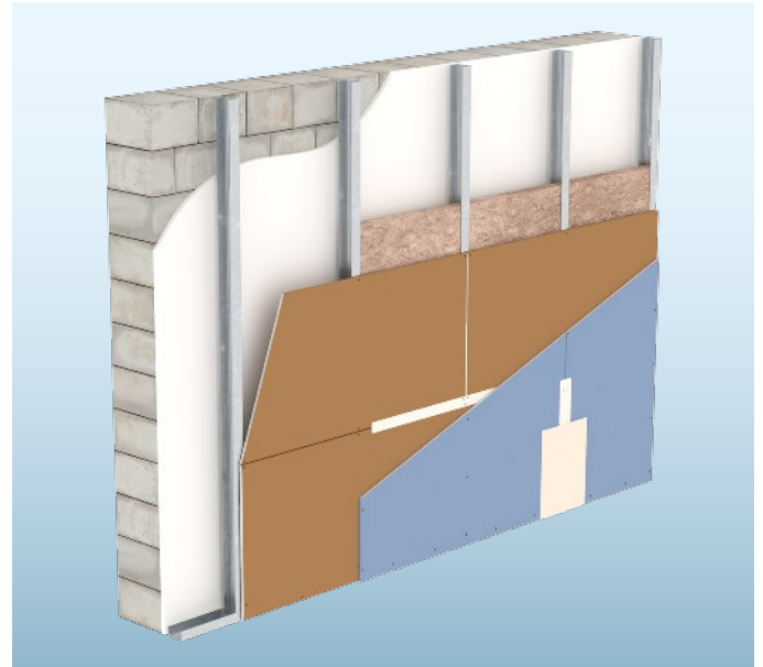
W626.de Vorsatzschale freistehend – Mehrlagig beplankt
