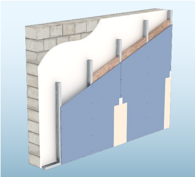
W625.de Vorsatzschale freistehend – Einlagig beplankt
