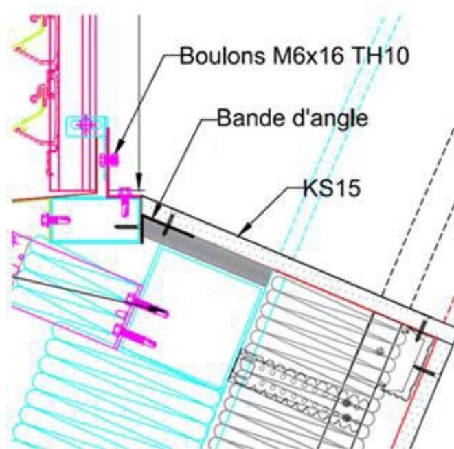
Jonction entre rampant et lucarne (chien-assis) sur toiture.
