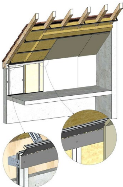
Jonction entre murs et rampants
