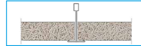
RAND A (SK-04)
