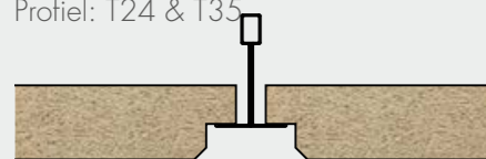
DOORZAKPANEEL - T24 Code: SK-06 T24 [E] Facet rondom Profiel: T24
