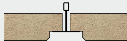
DOORZAKPANEEL - T35 Code: SK-06 T35 [E] Facet rondom Profiel: T35
