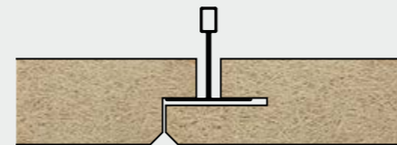
VERDEKT UITNEEMBAAR Code: VK-10 [D] Facet rondom Profiel: T35
