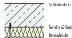
Schichtaufbau
