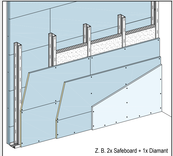
Strahlenschutzwand Safeboard + Diamant
