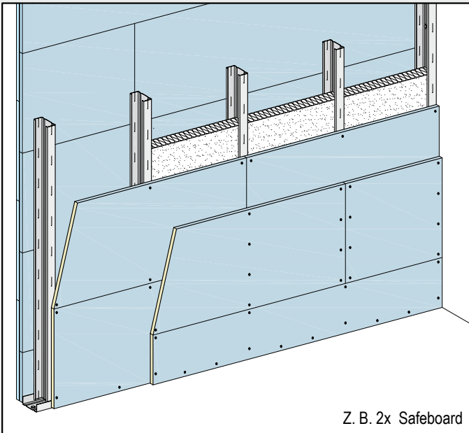
Strahlenschutzwand Safeboard
