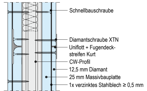
W118.de-WK2-VM10 Plattenstoß Vertikalschnitt
