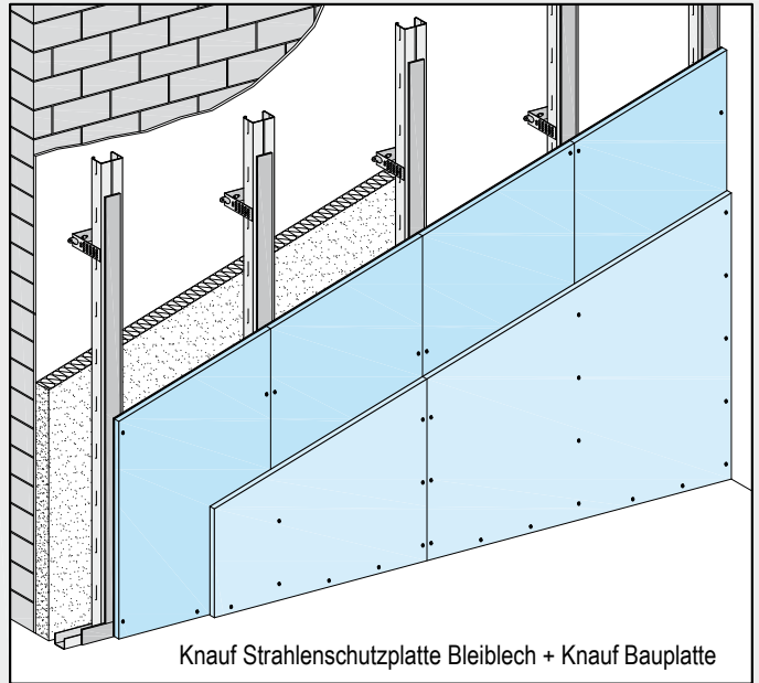
Knauf Strahlenschutzplatte Bleiblech
