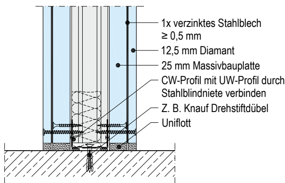
W118.de-WK2-VU10 Bodenanschluss
