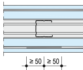
W118.de WK2 Einfachständer zweilagig beplankt
