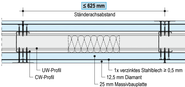
Schemazeichnung
