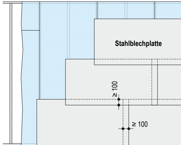
W118.de WK2 Einfachständer zweilagig beplankt
