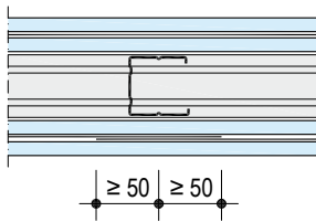
W118.de WK2 Einfachständer zweilagig beplankt
