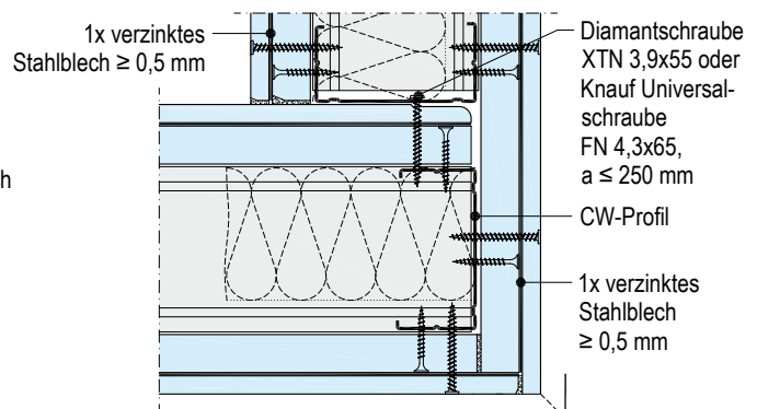
W118.de-WK2-D10 Ecke
