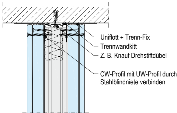
W118.de-WK2-VO10 Deckenanschluss
