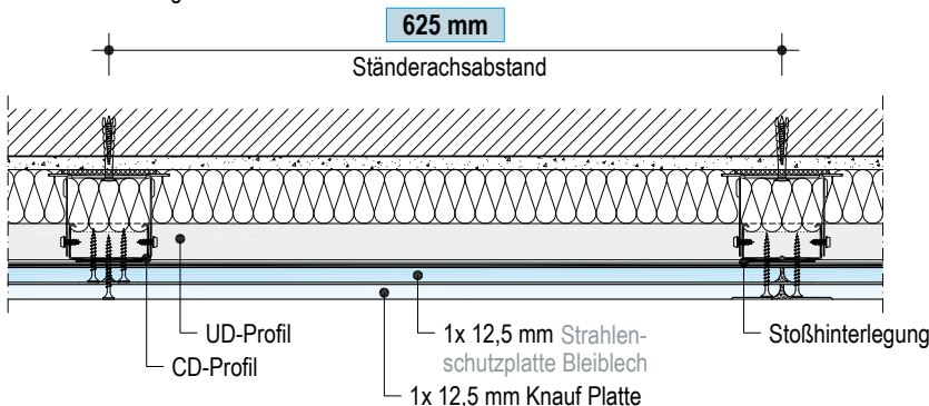
Schemazeichnung
