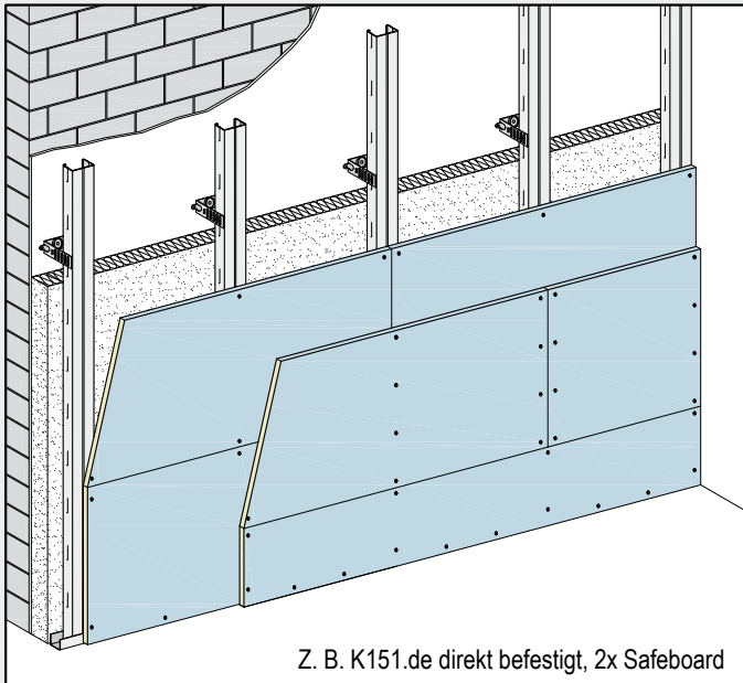
Strahlenschutz-Vorsatzschale Safeboard
