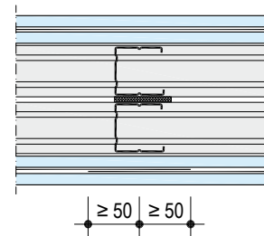
W119.de WK2 Doppelständer zweilagig beplankt
