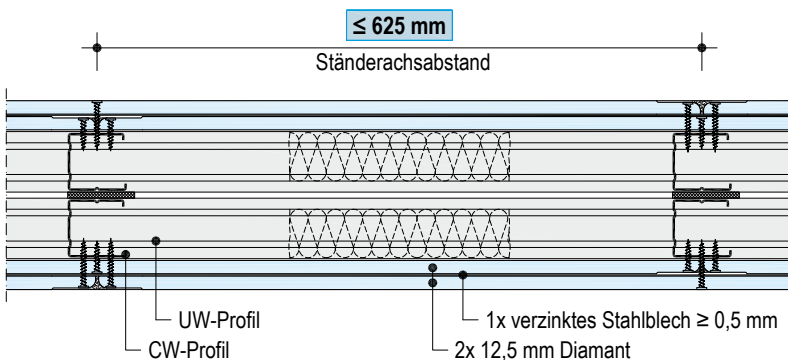
Schemazeichnung
