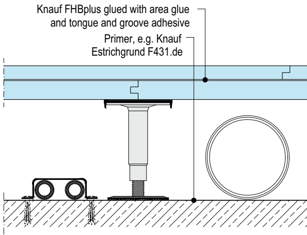
F182.de-V7 Partition on GIFAfloor FHBplus 32+18
