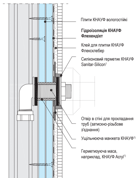
K435-V4 Прокладання труб
