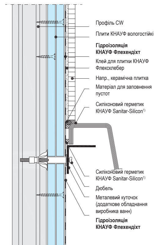
K435-V3 Кріплення ванни
