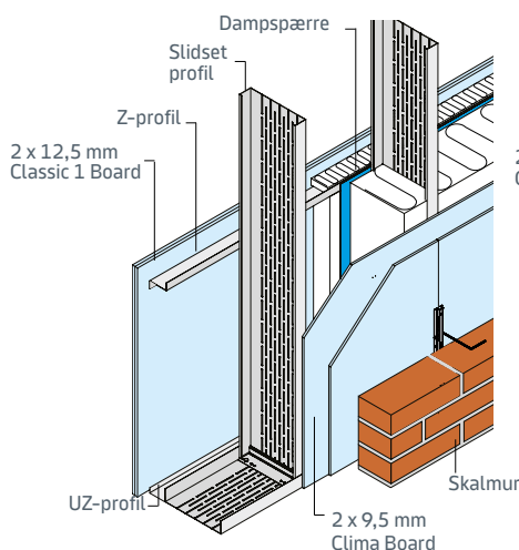
Eks. 1: Ydervæg med skalmur
