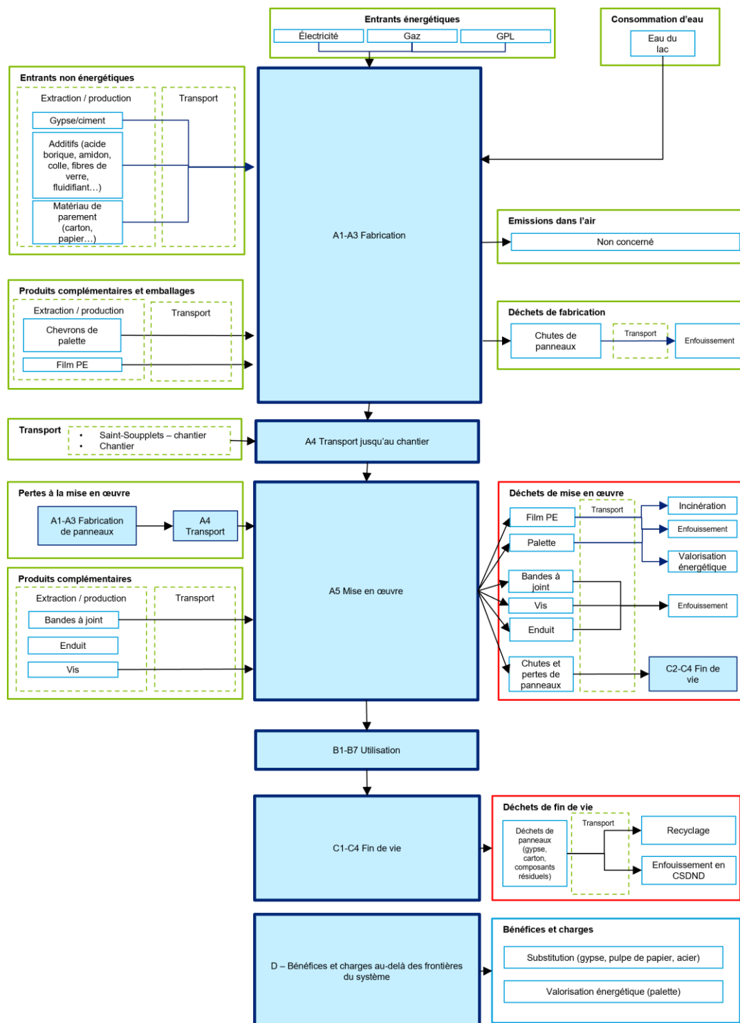
Diagramme du cycle de vie de la dalle Knauf Danoline Regula R 12.5mm
