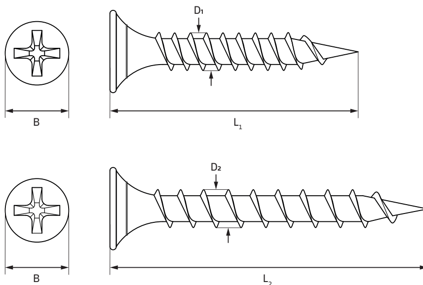
Tegning af hvide skruer til gipslofter til visualisering af mål i tabellen Produktdata
