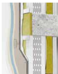
Jednostruka potkonstrukcija, uvučena montaža - uželježbljeni profili
