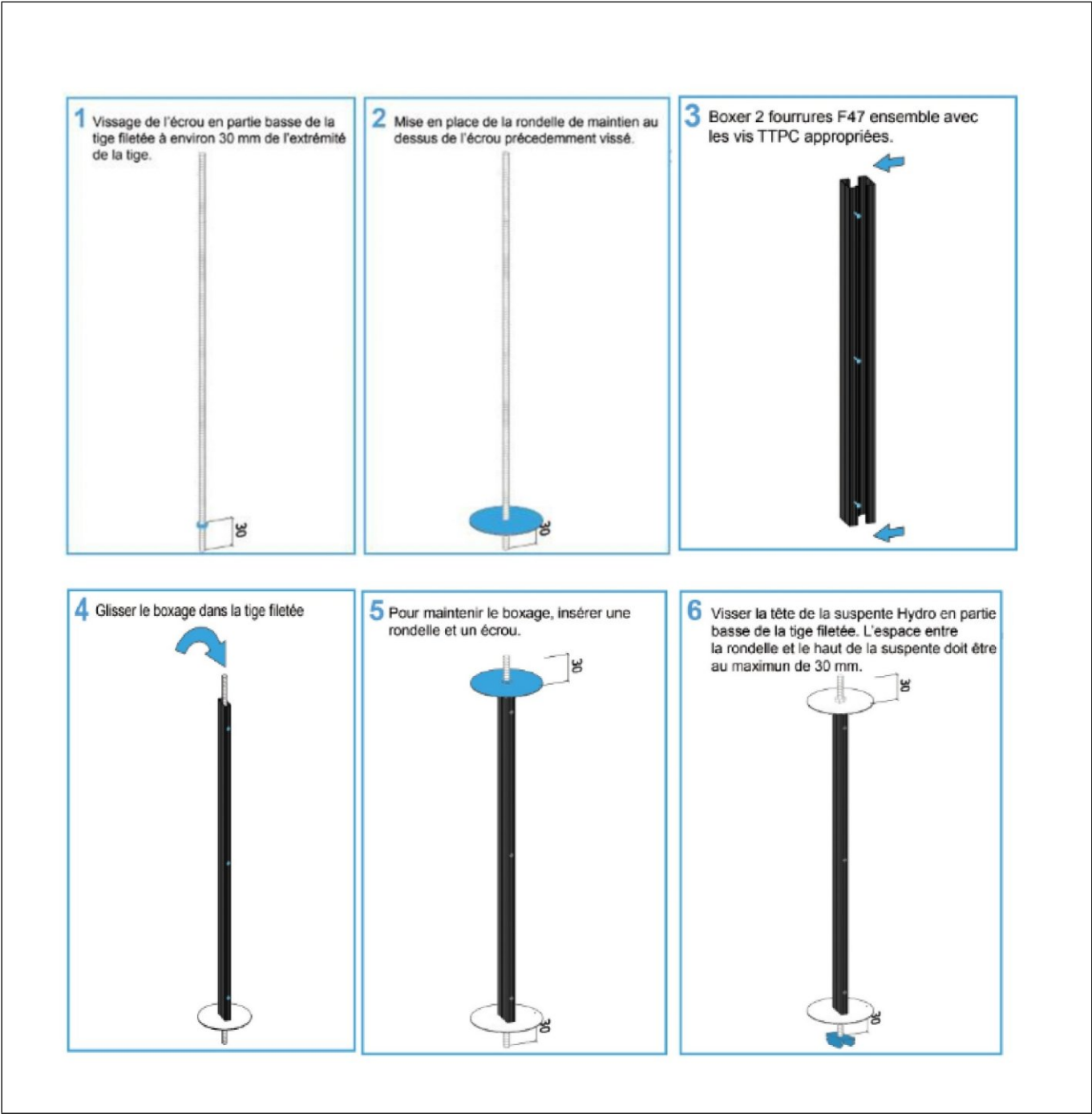
Figure 2 Mise en place du système de butonnage – Suspente Pivot F47 Hydro.
