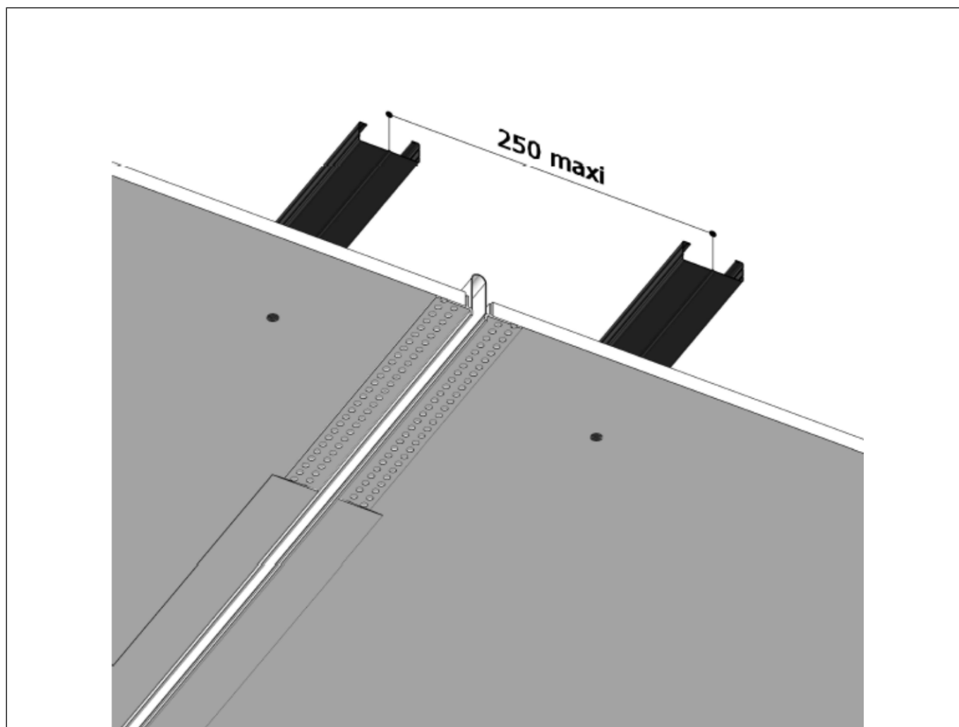
Figure 4 - Joint de fractionnement
