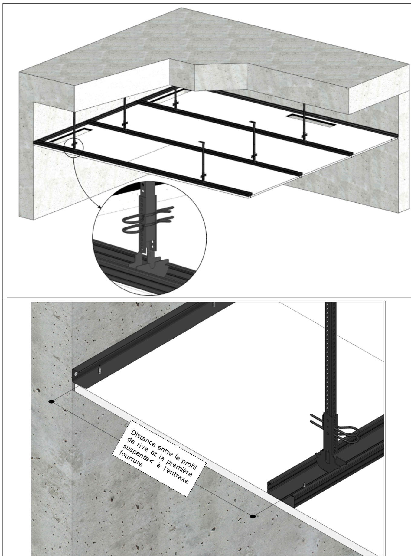
Figure 3 - Plafond extérieur Hydrodroof_Suspente réglable F47H à goupille parallèle à la fourrure F47
