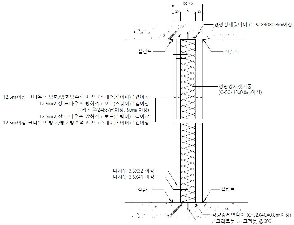
나. 수직 단면도
