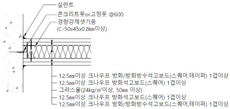
다. 벽 접합 상세도
