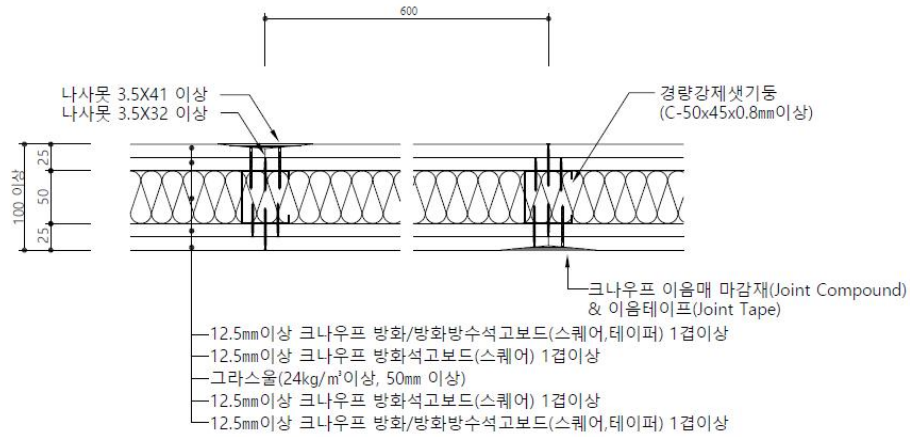
가. 수평 단면도
