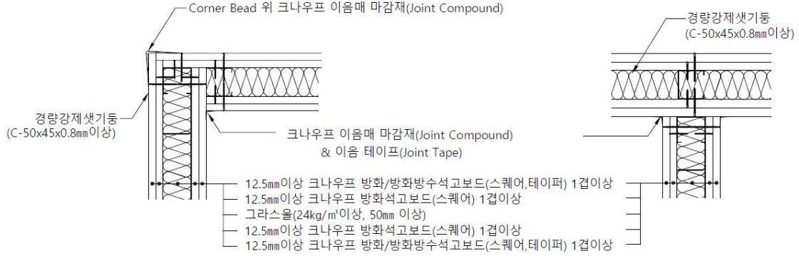
가. “ㄱ” 접합상세도
