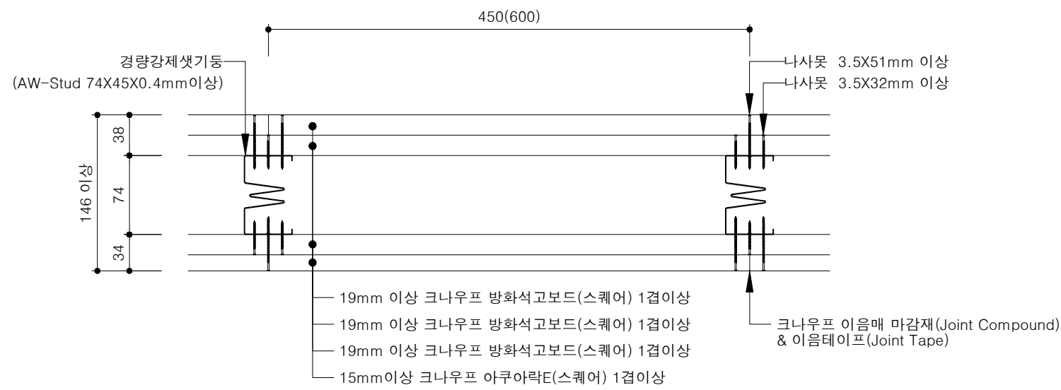
평면 상세도
