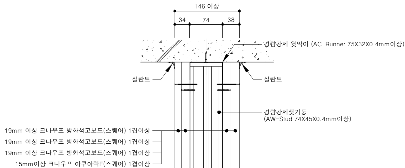
평면 상세도
