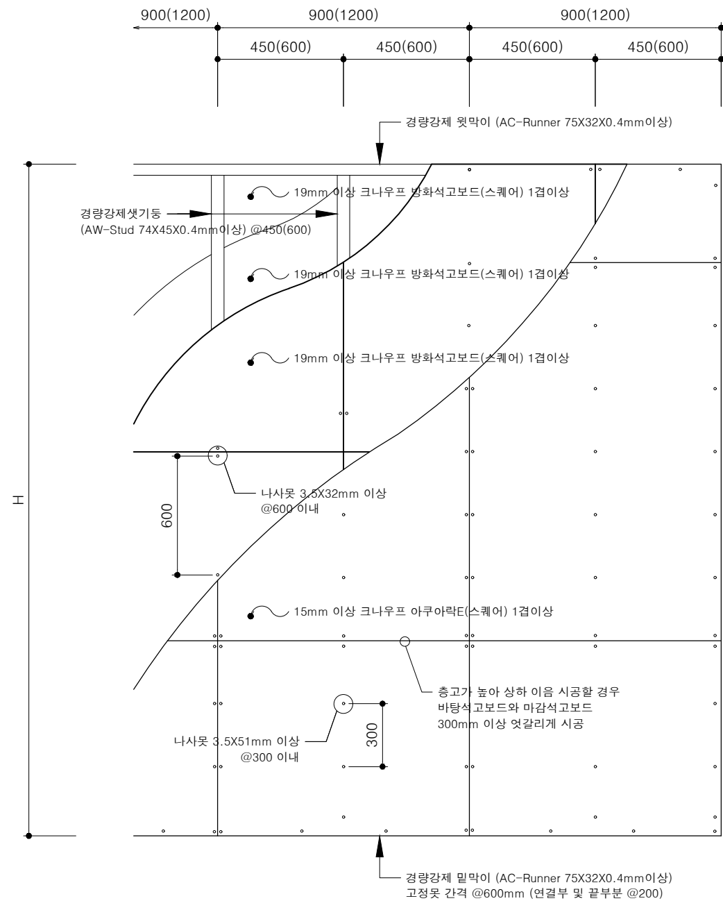
입면 상세도
