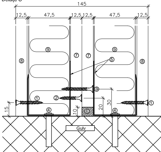
Detalje C
