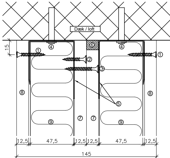
Detalje A
