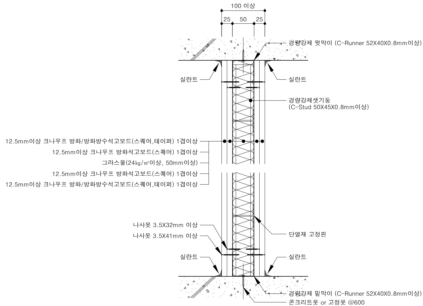
단면 상세도
