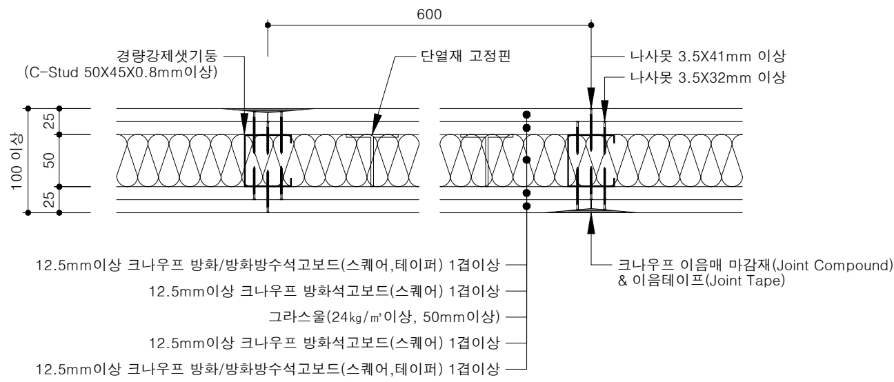
평면 상세도
