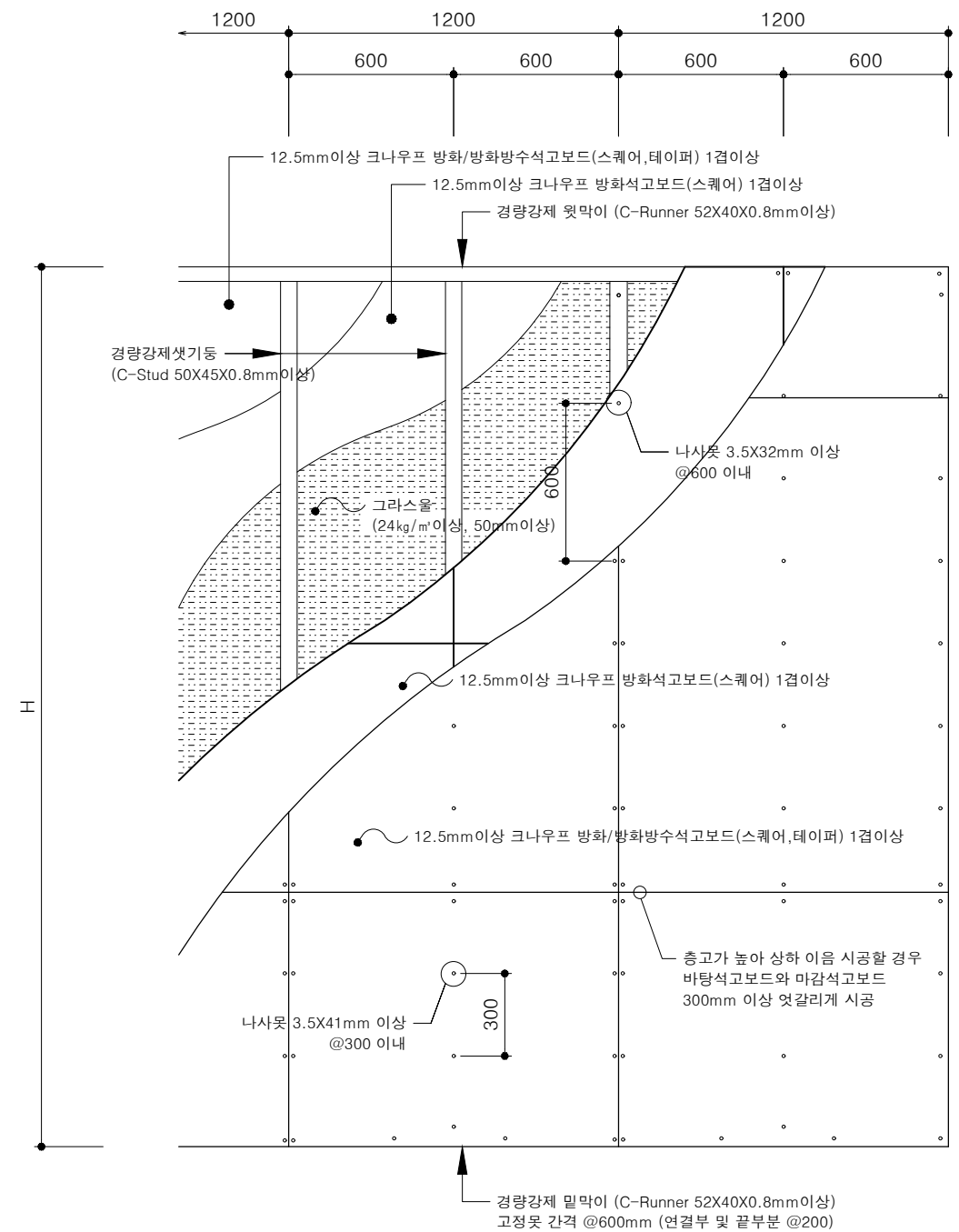
입면 상세도
