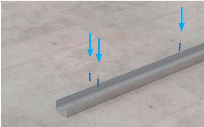
Bild 2: Knauf Pocket Kit Easy Höhenausgleich in UW-Profil einsetzen
