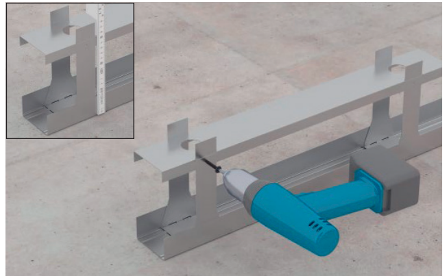
Bild 5: UW-Profil auf Knauf Pocket Kit Easy Höhenausgleich auflegen und ausrichten
