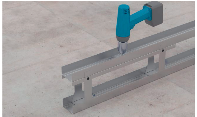
Bild 6: UW-Profil mit Knauf Pocket Kit Easy Höhenausgleich mittig fixieren
