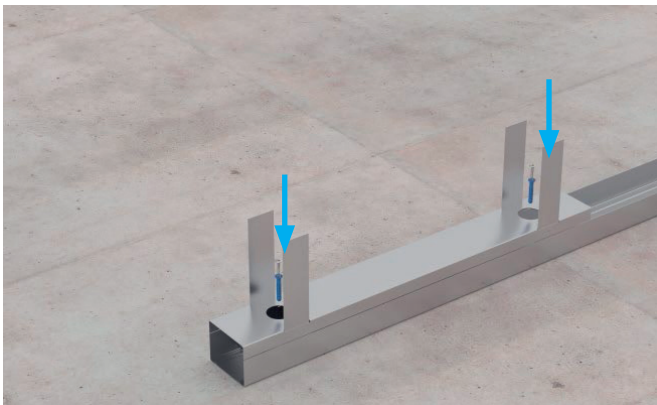
Bild 3: Höhenausgleich am Boden 2x durch die Löcher befestigen
