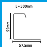
U vormige aansluitingsprofiel
