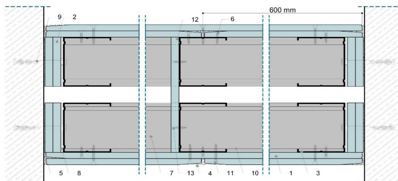
Фиг. 9.2 Странична връзка на стената с височина до 4 m
