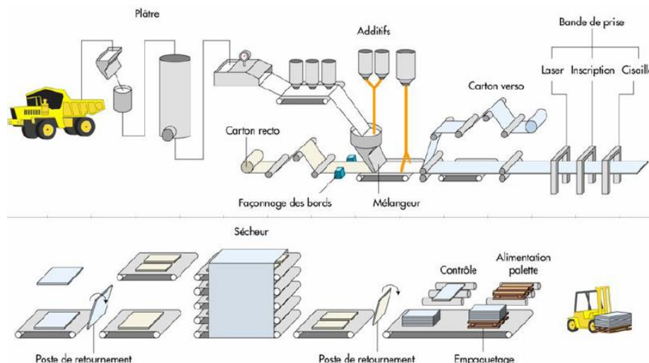
Schéma de production de la Knauf Danoline Plafond Perforé 12,5mm
