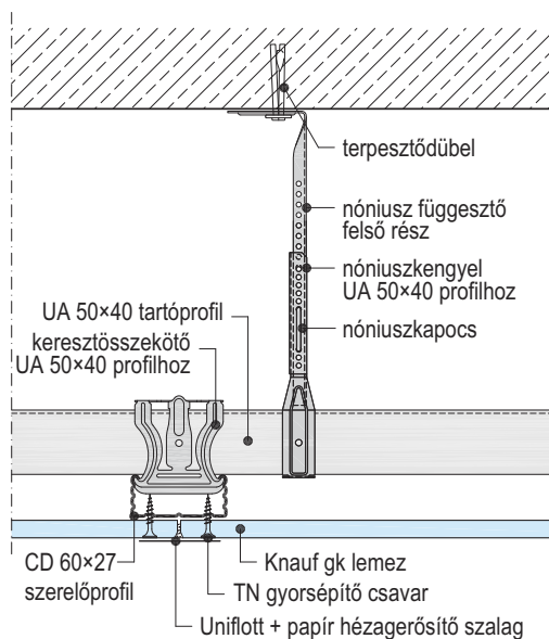
D116 - Kereszttillesztés
