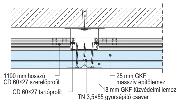
D112 - Mozgási hézag tűzvédelmi kivitelben
