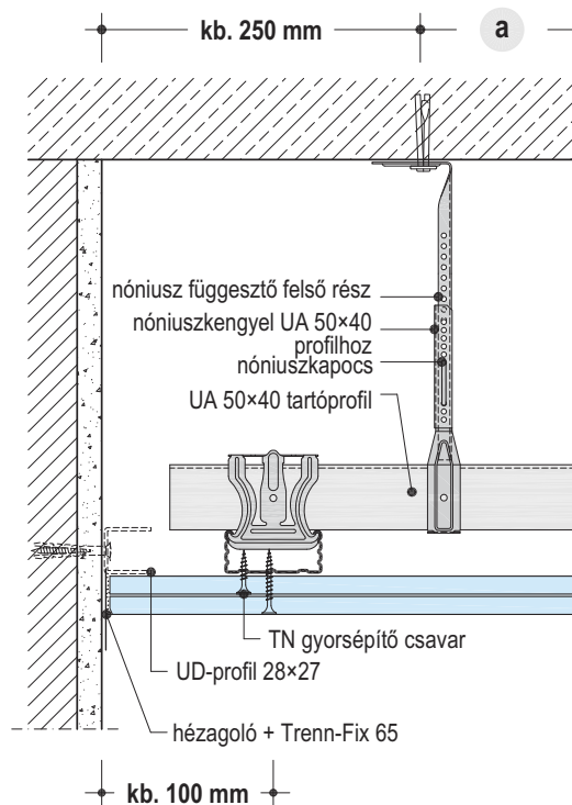
D116 - Kereszttillesztés
