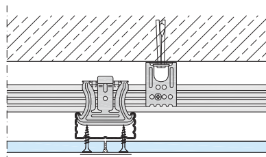
Kereszttillesztés
