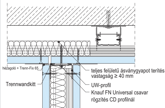
D112 - Csatlakozása álmennyezet-borításhoz
