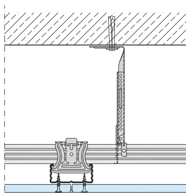
Kereszttillesztés
