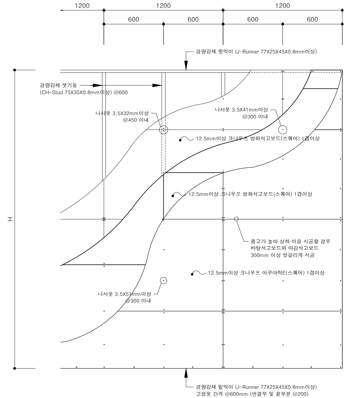
입면 상세도
