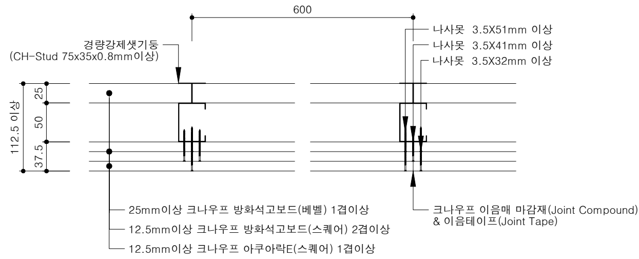
평면 상세도
