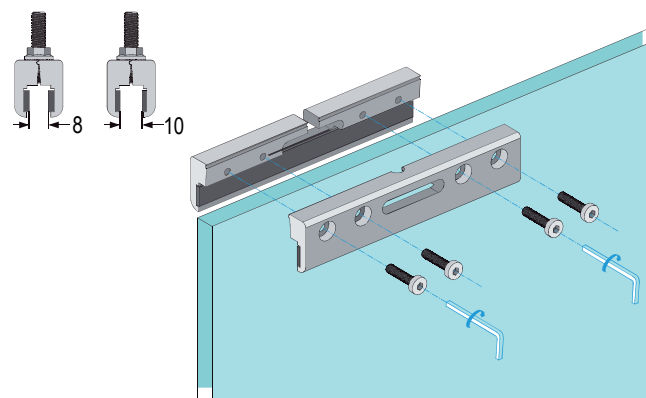
Bild 4: Klemmgummi vorbereiten
