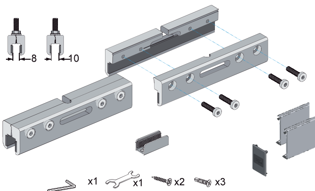
Bild 1: Inhalt Zubehörkarton
