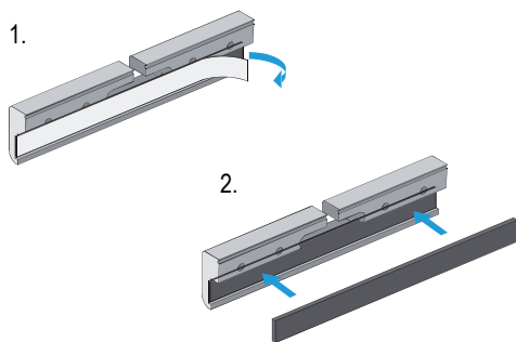
Bild 2: Klemmbacken vorbereiten
