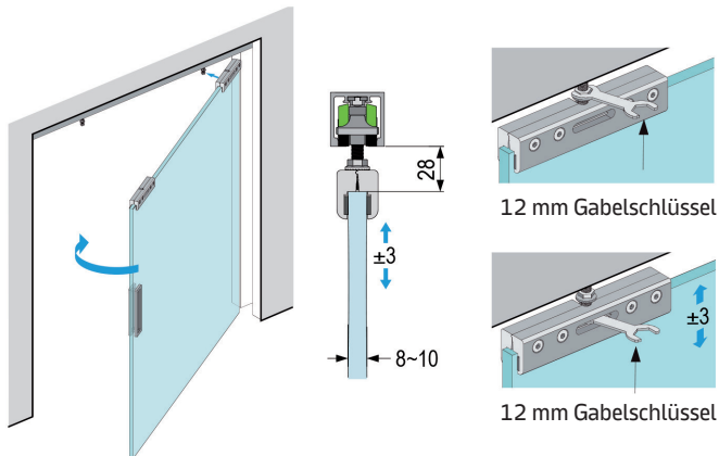
Bild 7: Türblatt montieren
