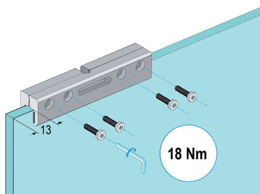
Bild 5: Klemmbacken positionieren
