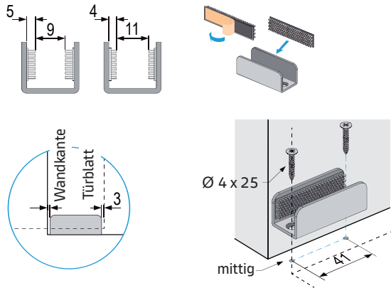
Bild 6: Mittelführung vorbereiten
