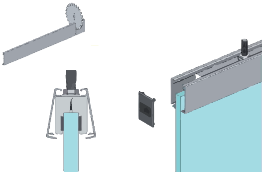
Bild 8: Blende Montieren
