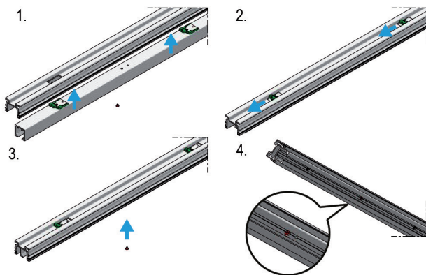
Bild 8: Laufschiene einsetzen
