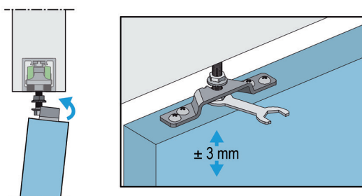
Bild 9: Tür einsetzen
