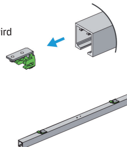
Bild 3: Laufschiene vorbereiten
