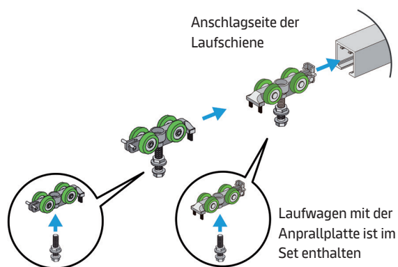
Bild 5: Laufwagen einsetzen
