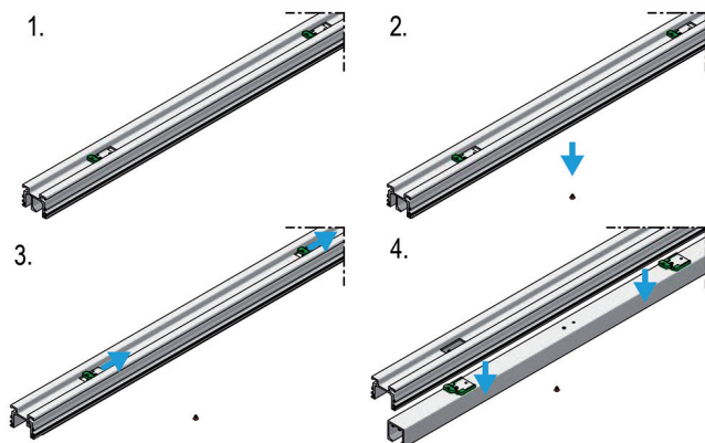
Bild 2: Laufschiene entnehmen
