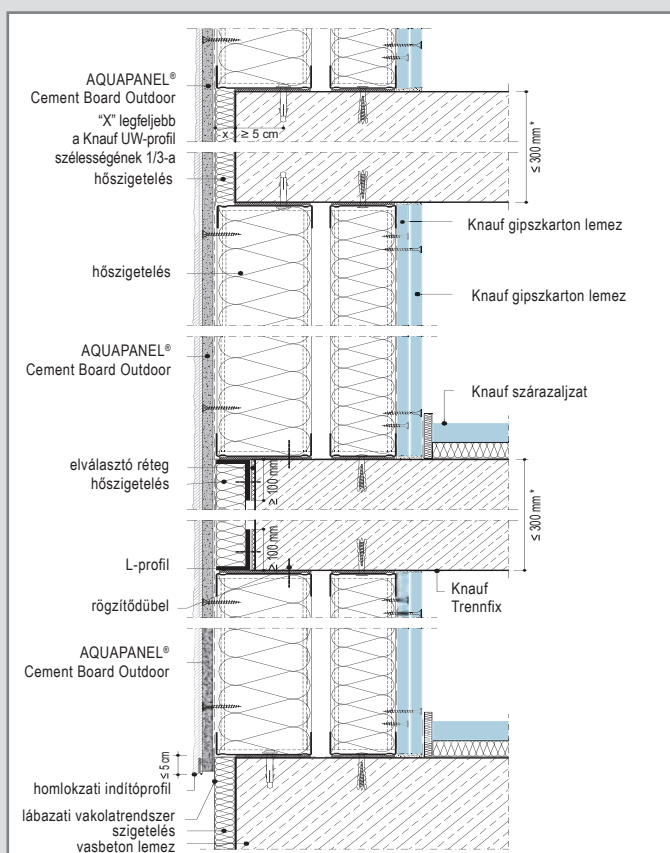
W388E-V1 Metszet
