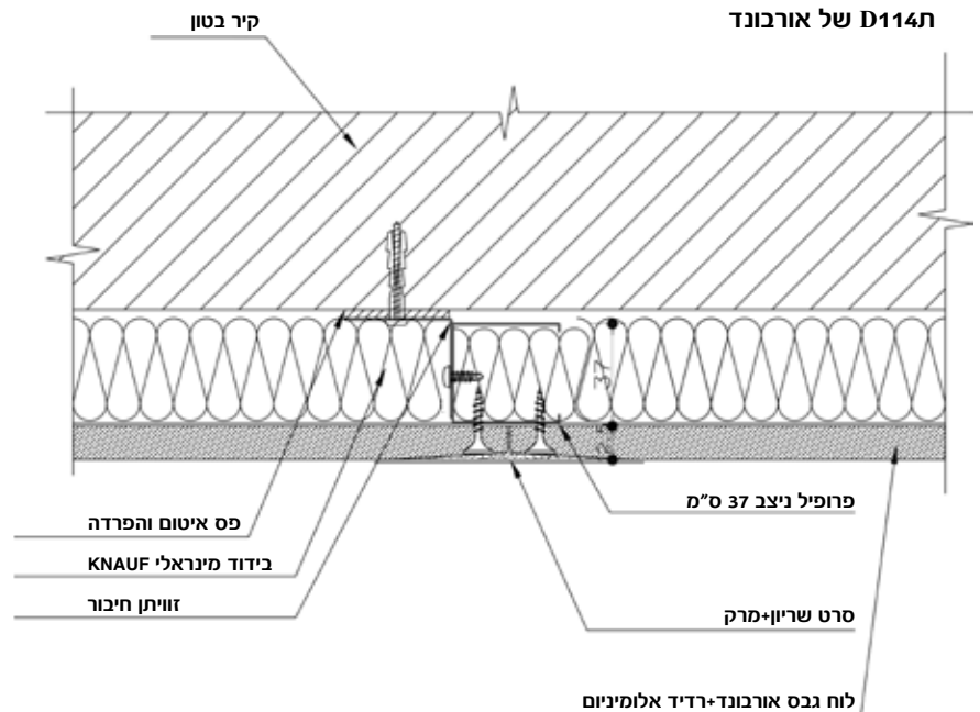
פרט חיפוי מרחב מוגן חתך אופקי
