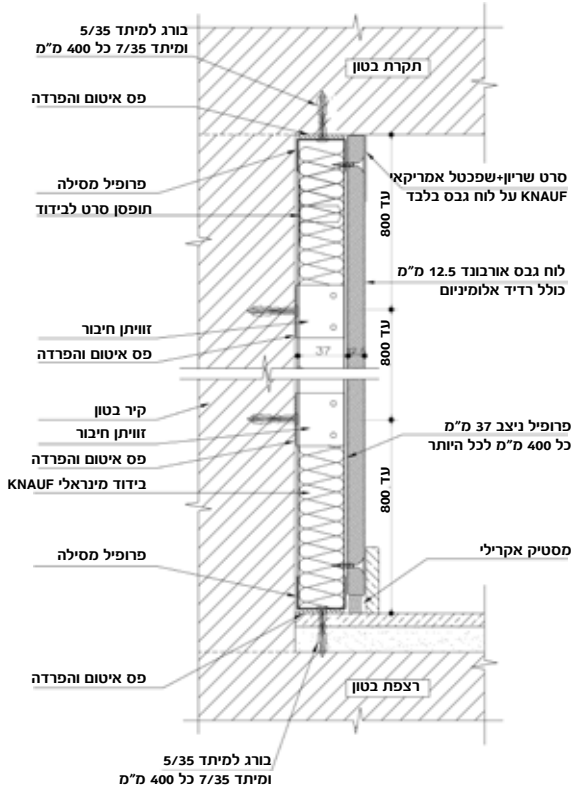
פרט חיפוי מרחב מוגן חתך אנכי
