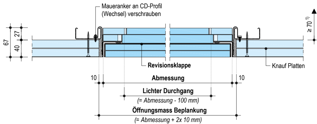
UP108.ch – V9, Schemaskizze EI 60
