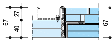
UP108.ch – V9.1, Schemaskizze EI 90
