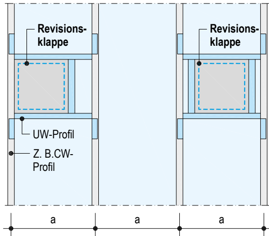
UP108.ch – V4 Beispiel Ständerachsenabstand a durchlaufend, System W628B.ch
