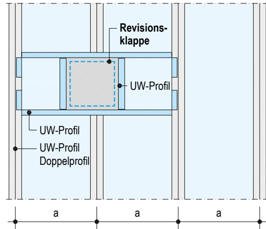
UP108.ch – V5 Beispiel Ständerachsenabstand a unterbrochen, System W629.ch
