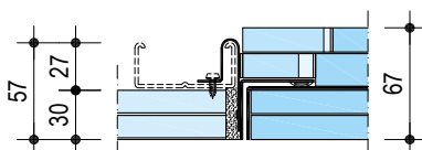
UP108.ch – V9, Schemaskizze EI 60
