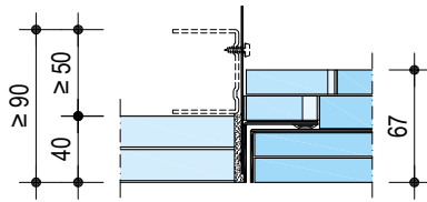
UP108.ch – V3, Schemaskizze EI 90
