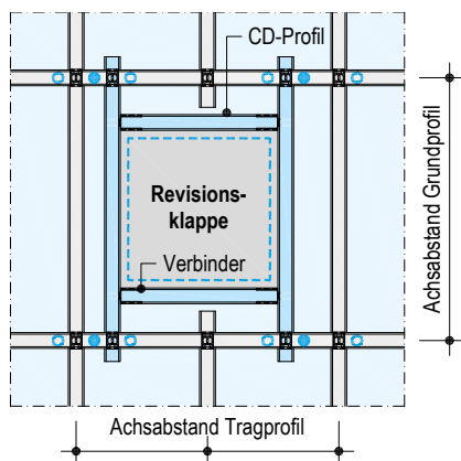
UP107.ch – V10, Schemaskizze Doppelter Profilrost (z.B D112.ch)
