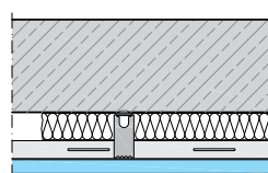
Spuštenu strop ovješenu direktnom elastičnom visilicom D112.hr
