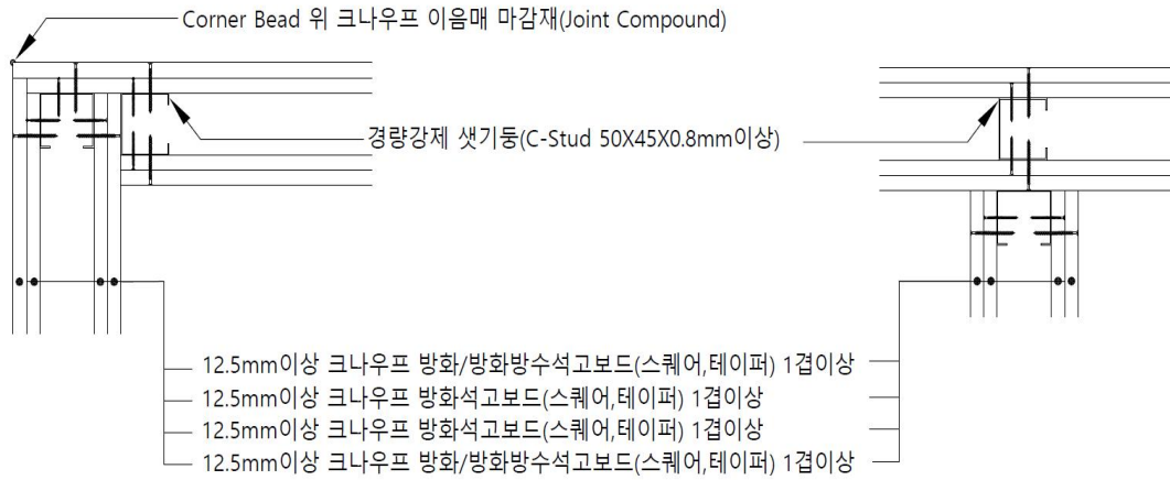
가. “ㄱ”접합상세도
