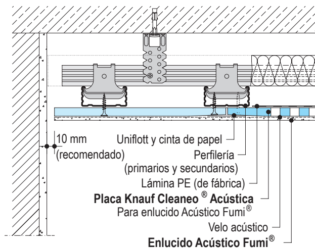
D126-D2.es Encuentro con tabique, junta con sombra y Friso
