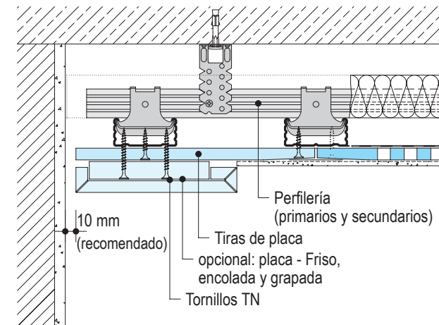
D126-D3.es Encuentro con tabique, junta con sombra y friso
