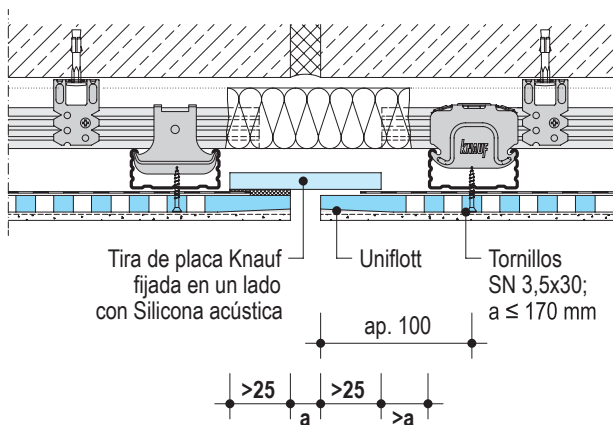
D126-C1.es Junta de dilatación
