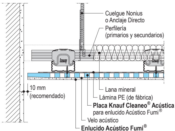
D126-D1.es Encuentro con tabique, junta con sombra
