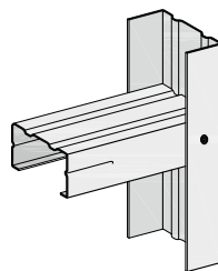
■ CW-Profile als Riegel
