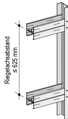
CW-Doppelprofile bevorzugte Variante bei Einbau Dämmschicht
