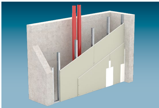
W628B.de Schachtwand mit Einfachprofil-Ständerwerk
