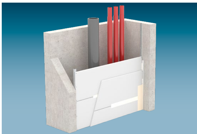
W630.de Schachtwand mit Riegelwerk
