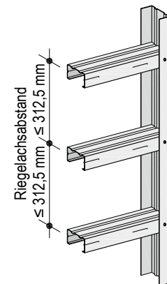
■ CW-Profile als Riegel
