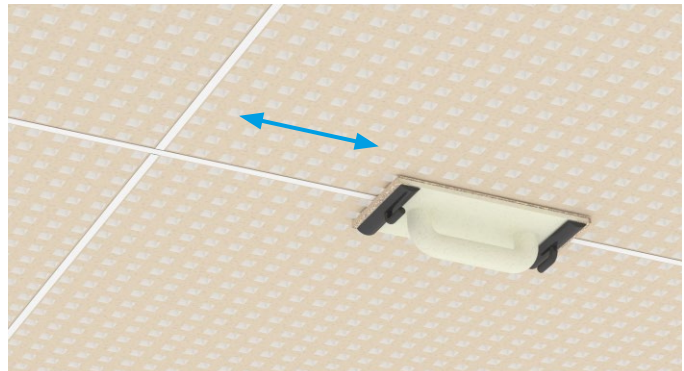
Bild 9: Egalisieren von Kleberstruktur
