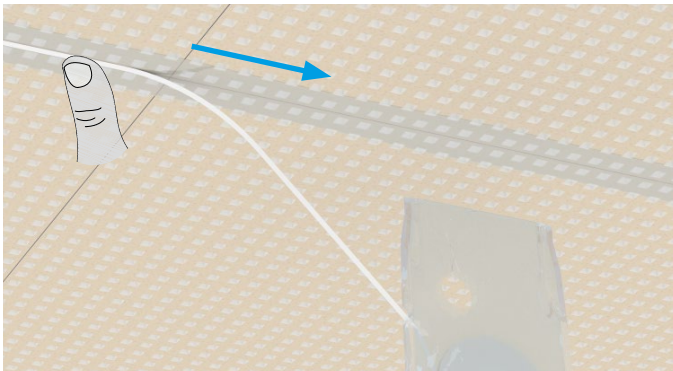
Bild 6: Cleaneo Tape über Fuge feststreifen
