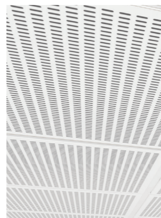
Tangent 14 x 4 mm, entraxe 10 et 20 mm Perforation: 21,4 %
