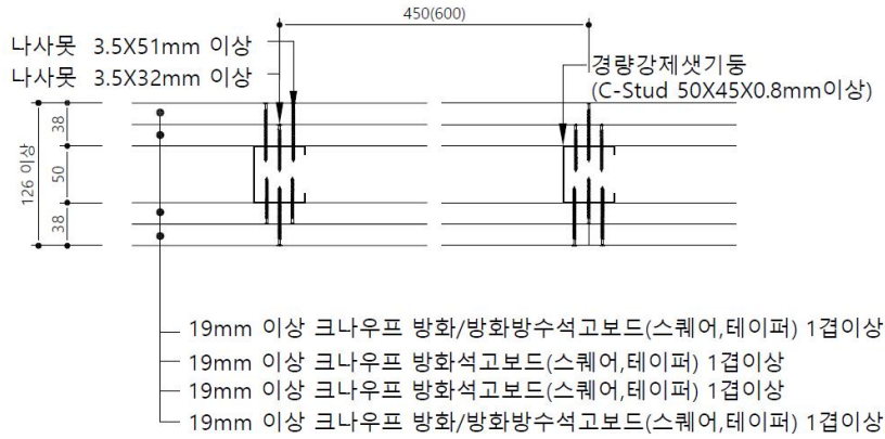
가. 수평 단면도
