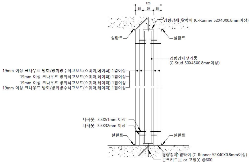
나. 수직 단면도
