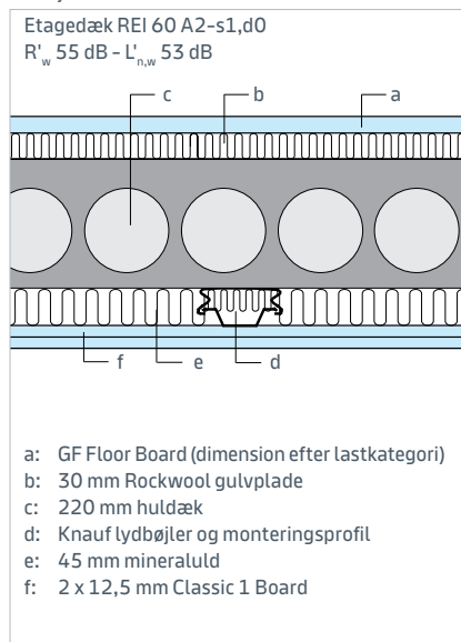
Detalje EB2
