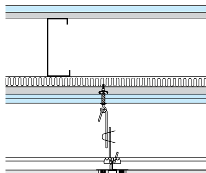
Nedhængt Knauf Danoline Systemloft. Fastgørelse i gipspladerne med Expandet Rosett.
