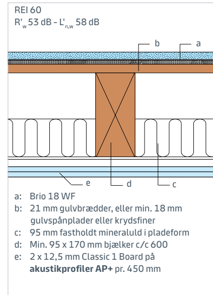
Detalje ET6
