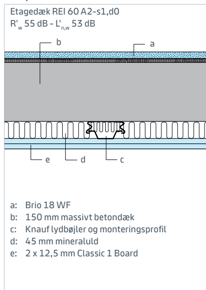
Detalje EB3
