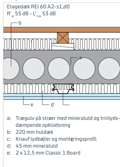
Detalje EB4
