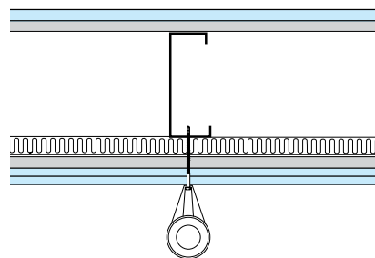
Ophæng af tunge genstande. Fastgørelse direkte i C-profil, (efter montage af gips).
