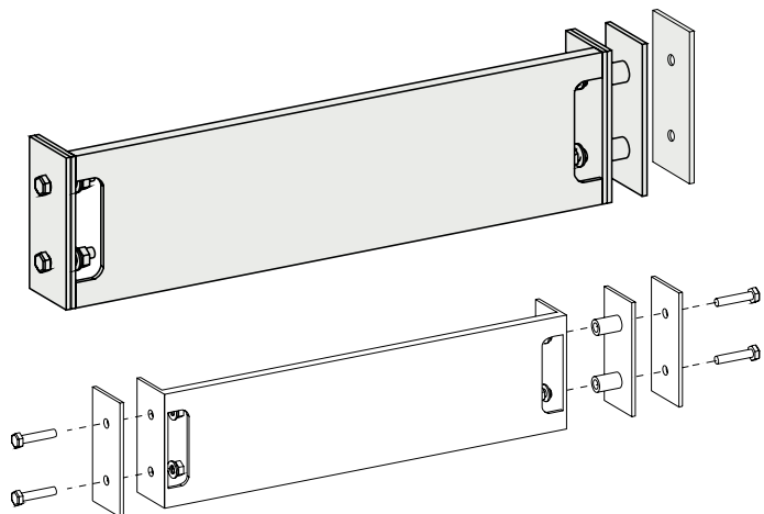
מותאם למרווח בין צירי ניצבים 600 מ"מ - מק"ט 2839103
