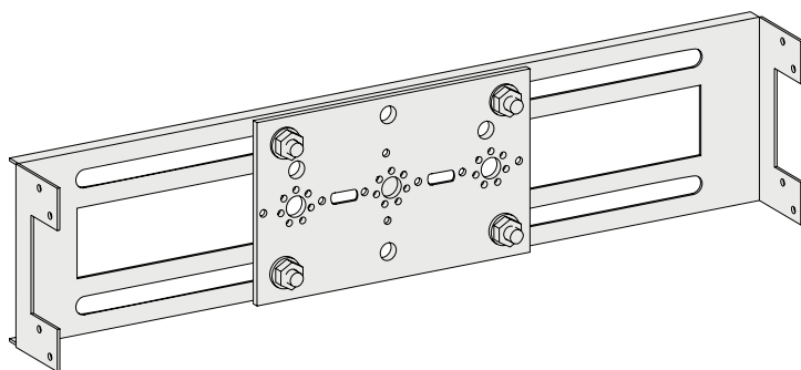
מותאם למרווח בין צירי ניצבים 600 מ"מ - מק"ט 2839098
