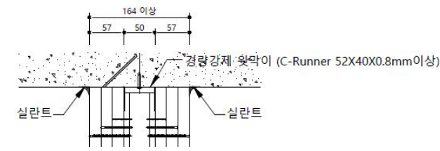
<상/하부 슬래브 접합부위 마감>
