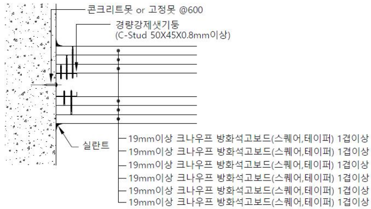
다. 벽 접합 상세도
