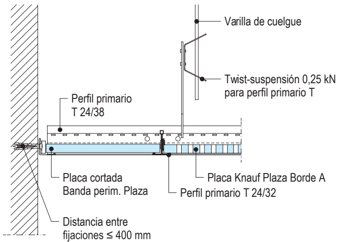
D145.es-D2 Encuentro con pared y perfil angular
