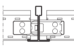
Perfil secundario T 24/32 (15/34) longitud 1200 mm
