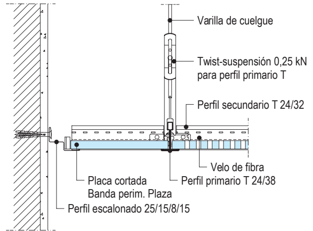
D146.es-A2 Encuentro con pared y perfil escalonado
