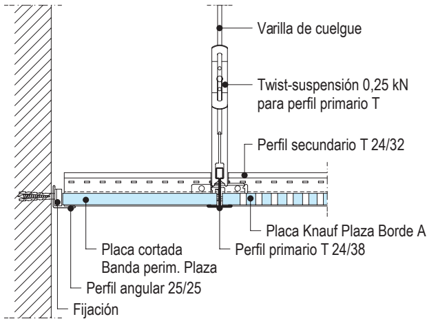
D146.es-A1 Banda perimetral con angular paralelo
