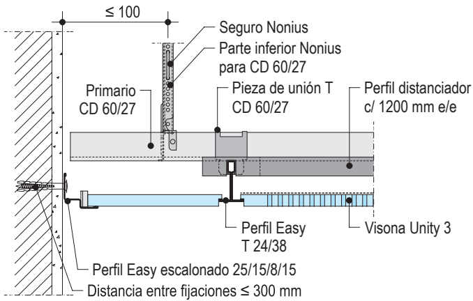
D144.es-B1 Sección longitudinal
