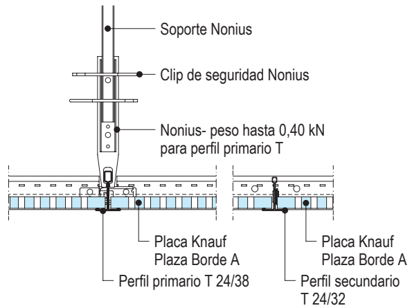
D146.es-B1 Encuentro entre perfil primario y secundario
