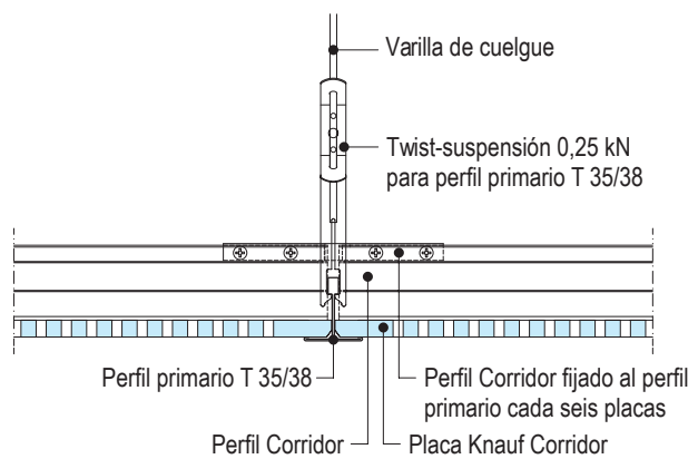
D148.es-A6 Empalme del techo para longitudes ≥ 2400 mm
