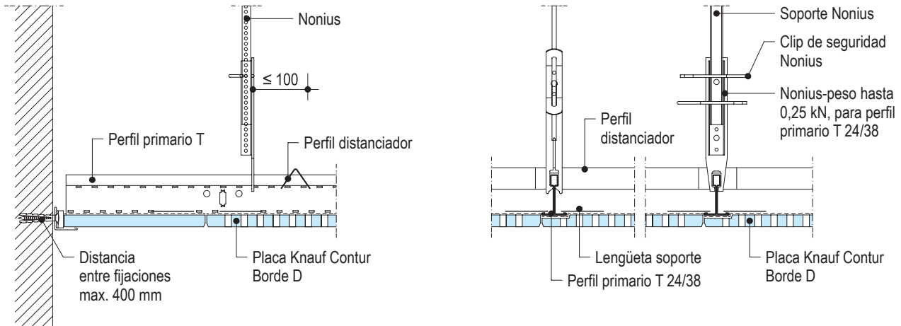
D147.es-D1 Banda perimetral con angular transversal al perfil
