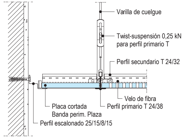
D145.es-B2 Encuentro entre perfil primario y secundario
