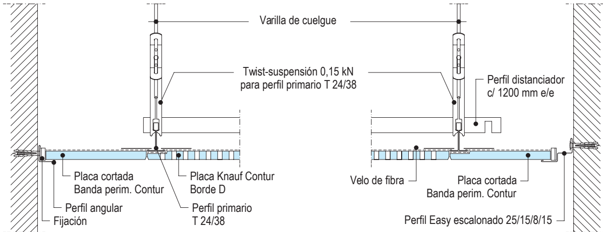
D147.es-A1 Banda perimetral con angular paralelo al perfil
