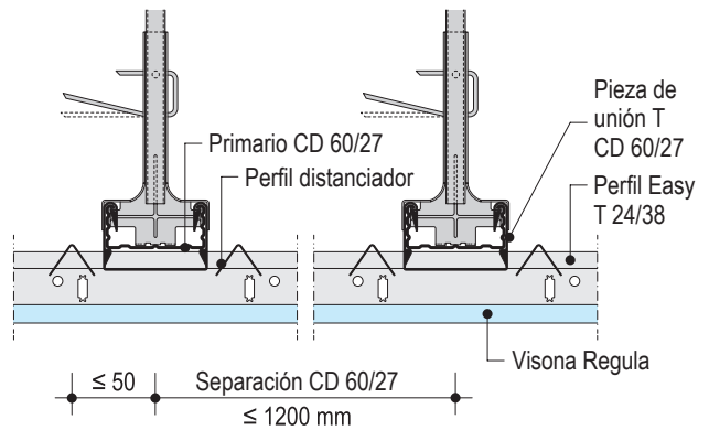
D144.es-C1 Sección transversal
