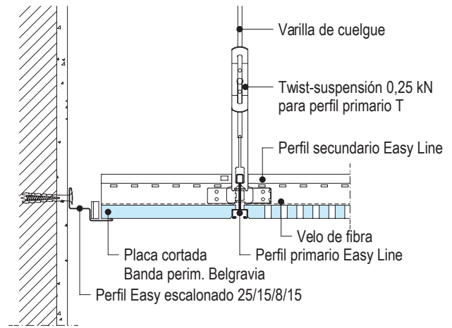
D145.es-B1 Encuentro entre primario y secundario
