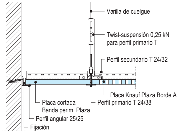
D145.es-A3 Banda perimetral con angular paralelo al perfil primario
