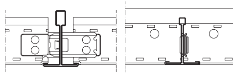
Perfil secundario T 24/32 (15/34) longitud 1200 mm
