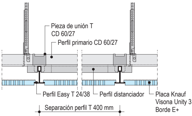
D144.es-B1 Sección longitudinal
