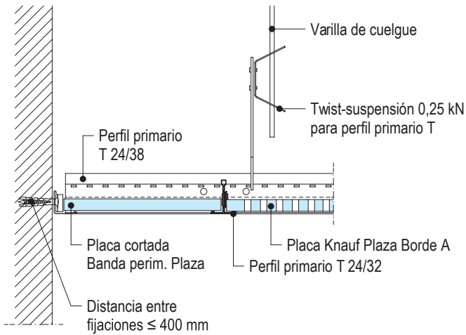
D146.es-D1 Banda perimetral con angular transversal
