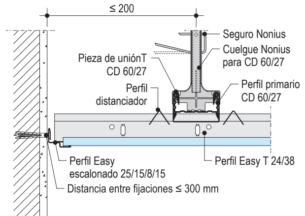
D144.es-C1 Sección transversal
