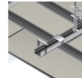
Alternatieve ophanging met AQUAPANEL® directafhangers
