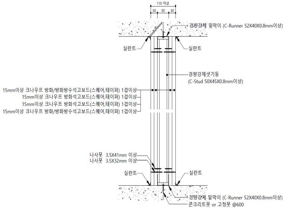
나. 수직 단면도
