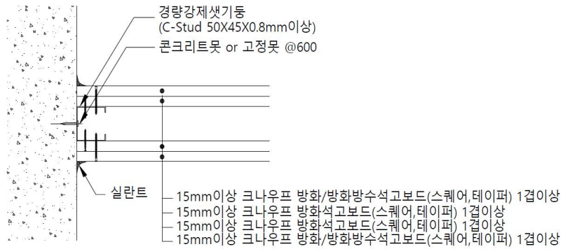
다. 벽 접합 상세도
