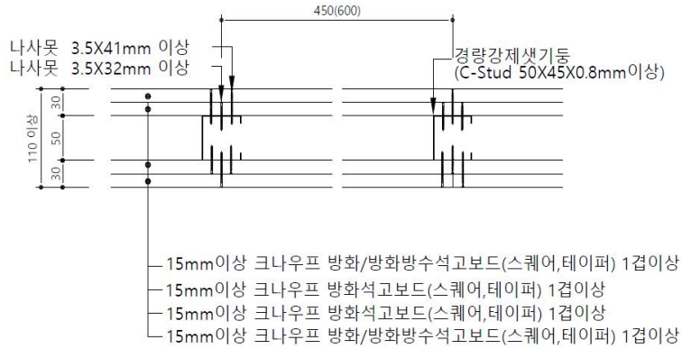
가. 수평 단면도
