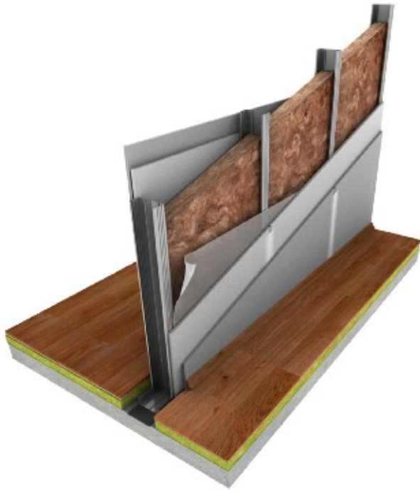
Perete de compartimentare din gips-carton ex: KNAUF W112
