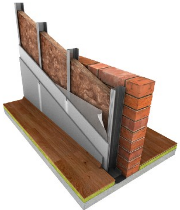
Perete portant placat cu gips-carton pe structura independentă ex: KNAUF W626
