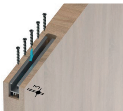
Bild 12: Schiene mit Schrauben 4 x 38 mm am Türblatt befestigen
