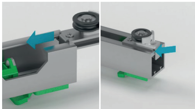
Bild 7: Stopper mit langer Führungsschiene in die Laufschiene
