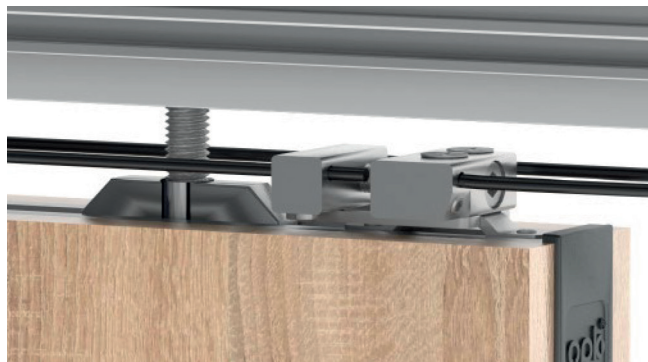
Bild 27: Seil in den Spannklotz ziehen
