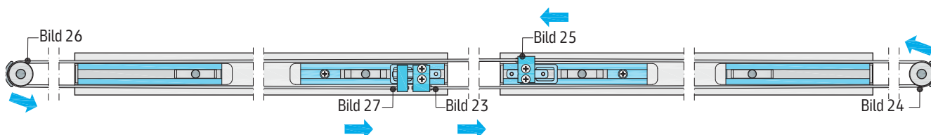
Bild 22: Übersicht Seilführung
