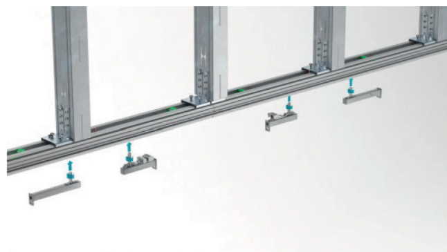
Bild 13: Einschrauben der Aufhängungen
