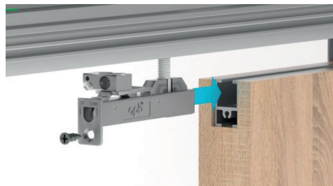
Bild 18: Aufhängung in die Schiene der Türe schieben
