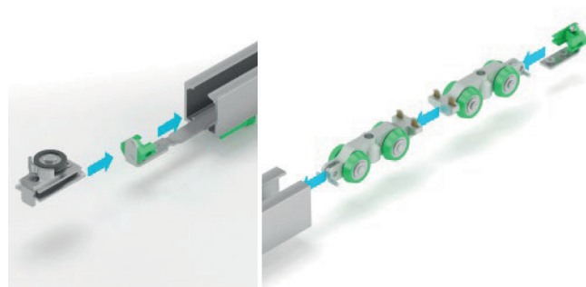
Bild 9: Bestücken der zweiten Laufschiene
