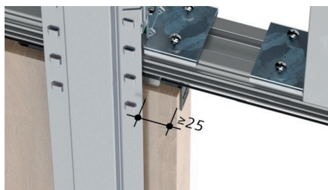
Bild 32: Türe bei Vollversenkung entspricht das Mass 25 mm
