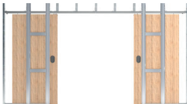
Bild 21: Montieren der zweiten Tür analog der ersten
