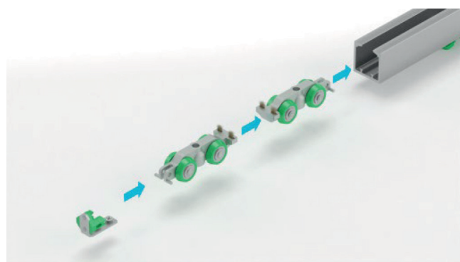
Bild 8: Laufschiene bestücken
