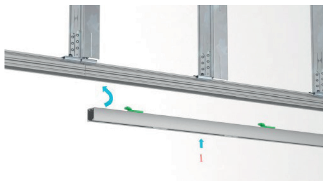
Bild 10: Einsetzen der Laufschiene
