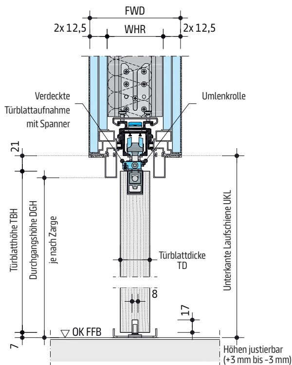
Bild 3: Darstellung Vertikalschnitt – Synchronöffnung
