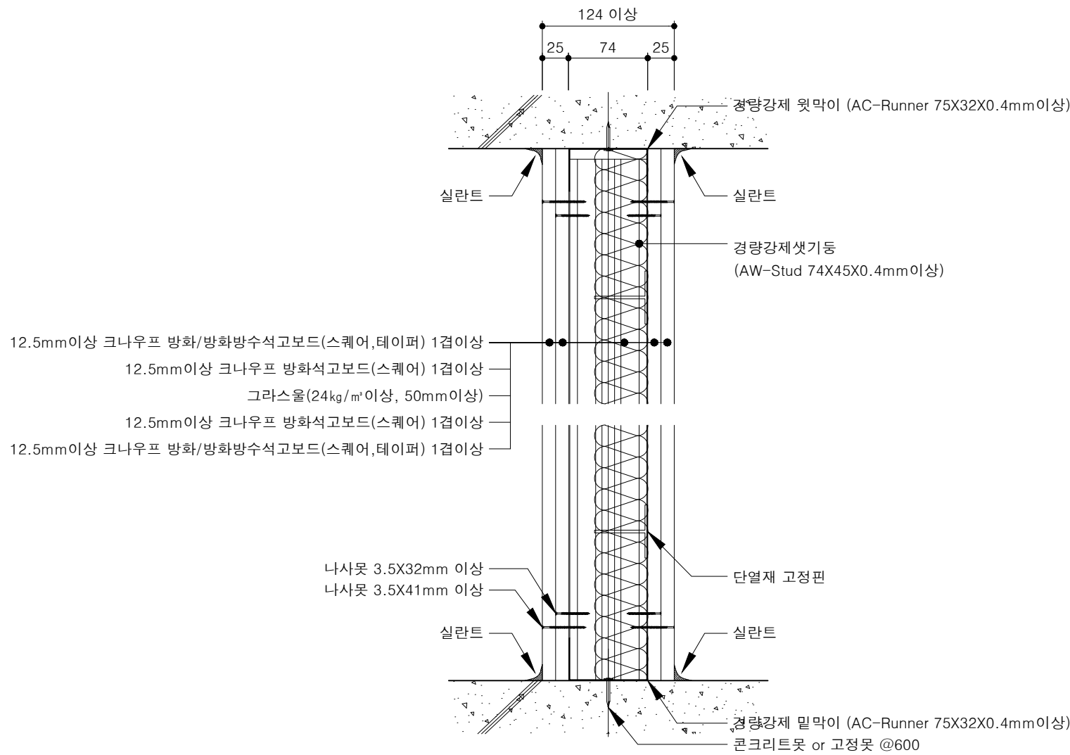
단면 상세도
