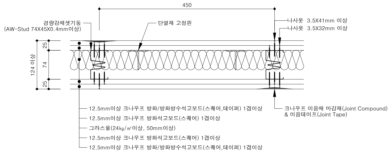
평면 상세도
