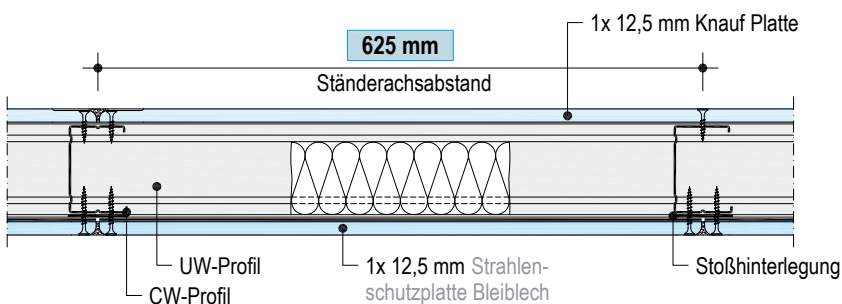
Schemazeichnung
