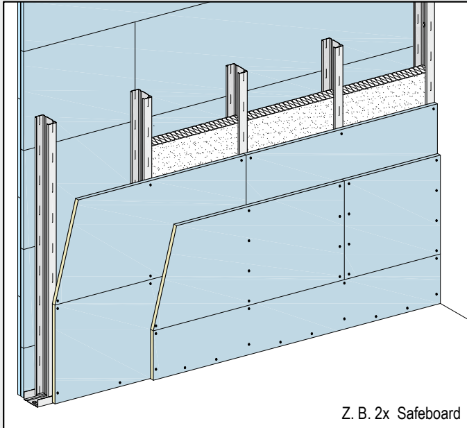
Strahlenschutzwand Safeboard
