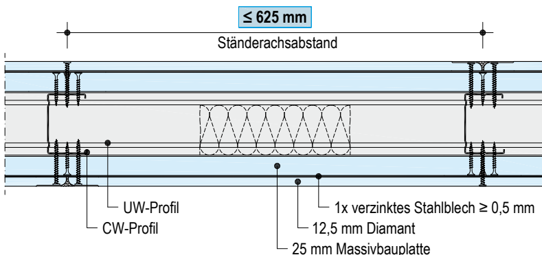
Schemazeichnung
