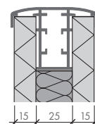
Baffle Line com moldura em todos os lados
