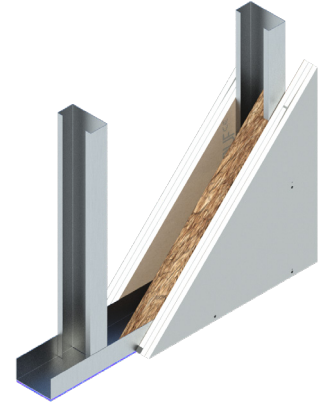
Principskitse
