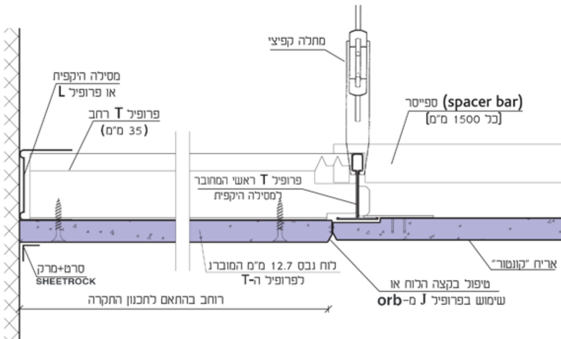
חתך דרך פרופיל ה T (צד ימין)
