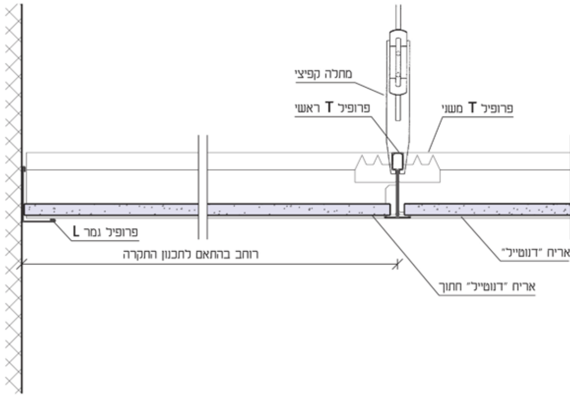
אריח דנוטייל DANOTILE 600 קנ"מ 1:2.5
