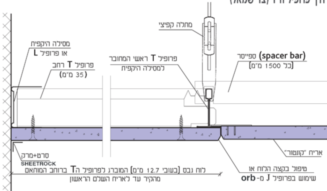
חתך דרך פרופיל ה T (צד שמאל)
