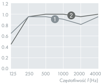
1 HERADESIGN® Fine plus 25+25 mm TKH 200 mm \alpha_w 0.90 (L) NRC = 0.90 Klasa pochłaniania dźwięku A
