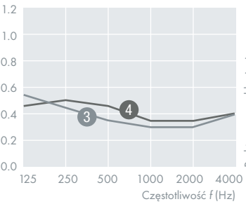
3 HERADESIGN® Micro plus 25+25 mm TKH 200 mm \alpha_w 0.35 (L) NRC = 0.35 Klasa pochłaniania dźwięku D
