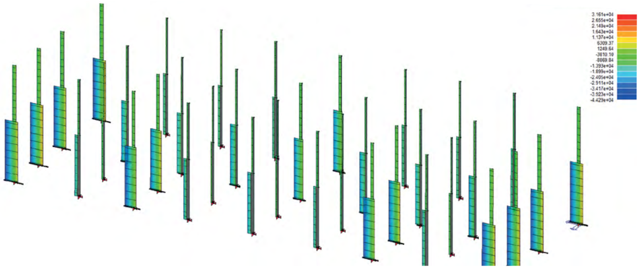
RISULTATI: Involuppo Sforzo Normale Fx - Pilastri (daN)
